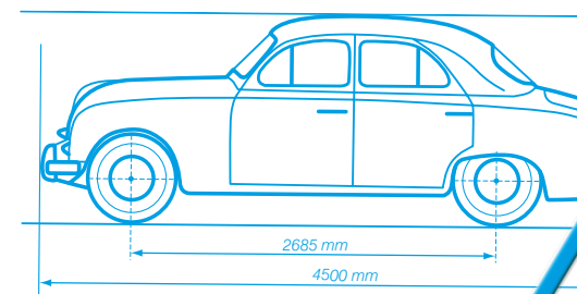
technický výkres a podrobné technické parametre vozidla
