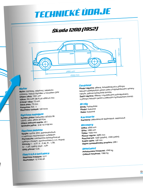
technický výkres a podrobné technické parametre vozidla
